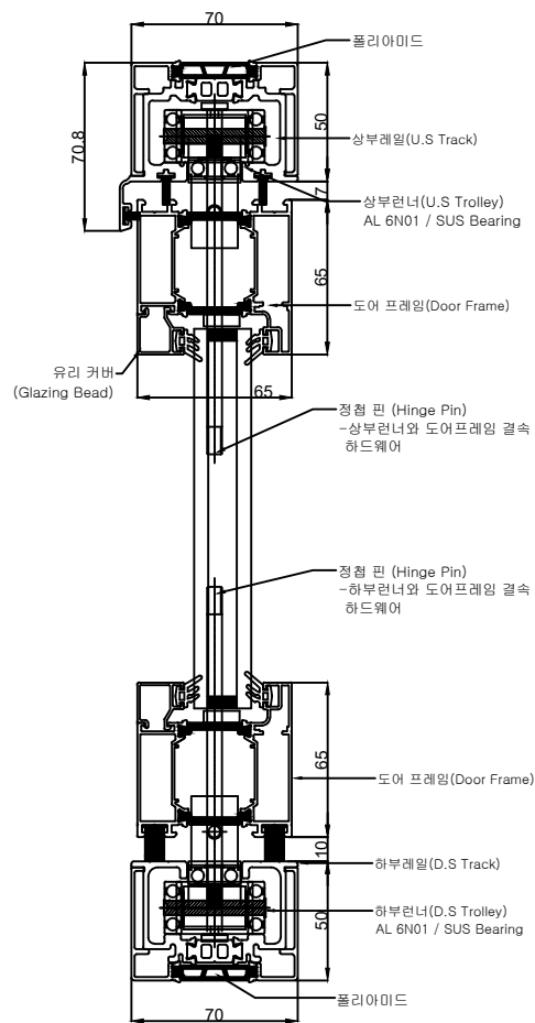
② SCALE none 단면도
